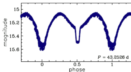
Figura 5: Curva de magnitud con respecto a fase de un sistema binario eclipsante tipo Algol en el que una estrella posee un disco de acreción. Se observa como el eclipse primario es más largo que el secundario.
