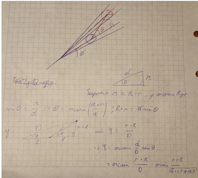
Figura 18: Demostración manual del ángulo de separación entre los planos de observación de dos estrellas de un sistema binario para que el observador las considere eclipsantes.
