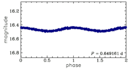
Figura 12: Curva de magnitud con respecto a fase de una ceféida clásica oscilando en el segundo armónico. La amplitud de la oscilación es muy pequeña, y la oscilación en sí es prácticamente sinusoidal.
